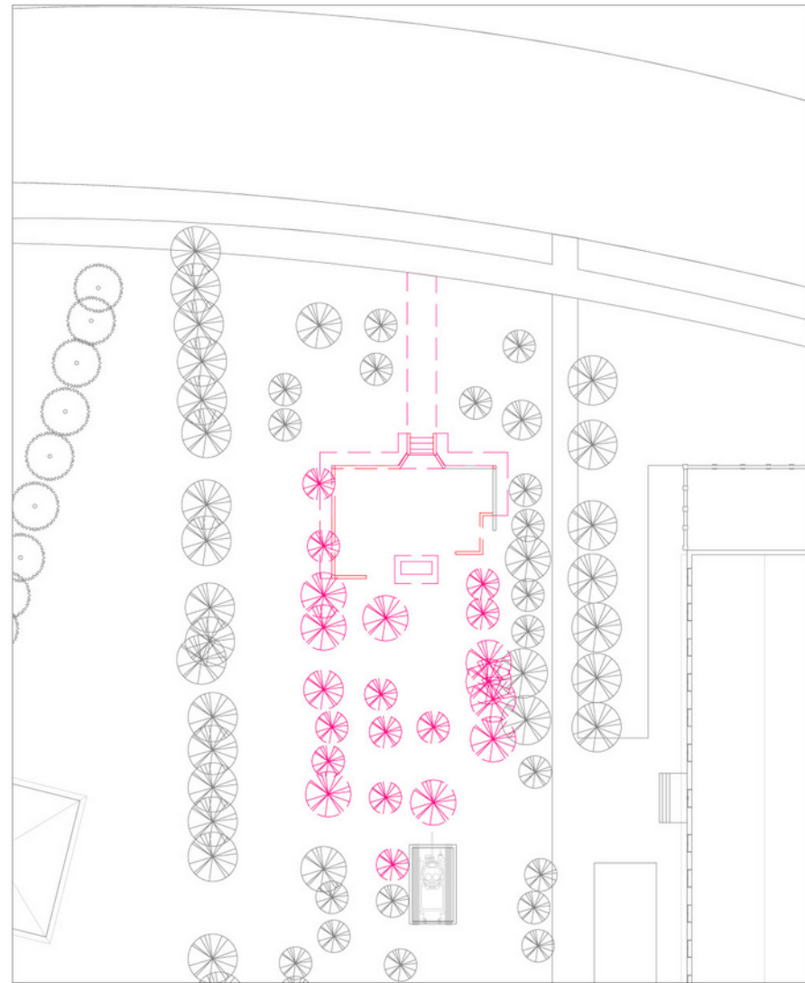
План демонтажа
